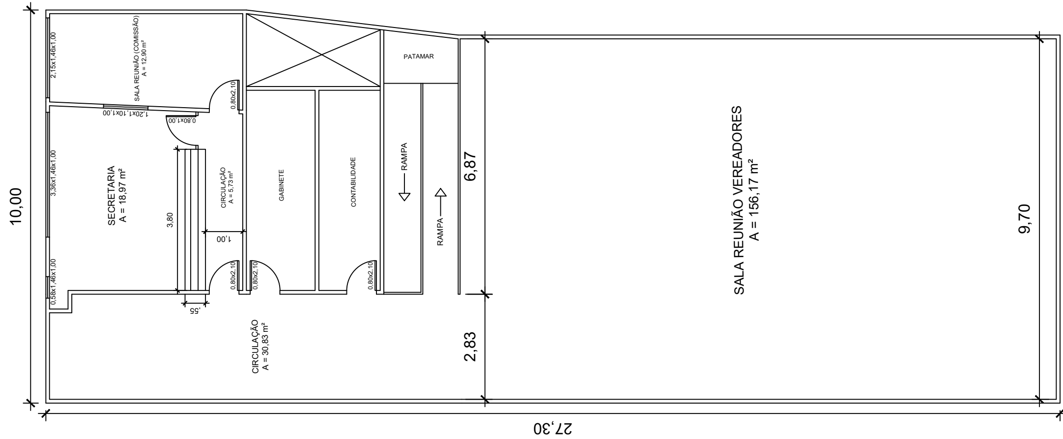
PLANTA BAIXA 1º PAVIMENTO ESC. 1:100
